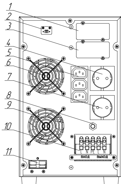
Рисунок 3в. Компоненты задней панели ИБП Штиль ST1103TL
