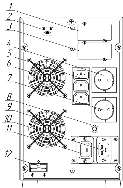
Рисунок 3б. Компоненты задней панели ИБП Штиль ST1102SL, ST1102L, ST1103SL и ST1103L
